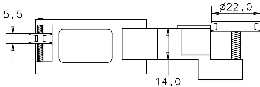
Seitenansicht von links side view left
