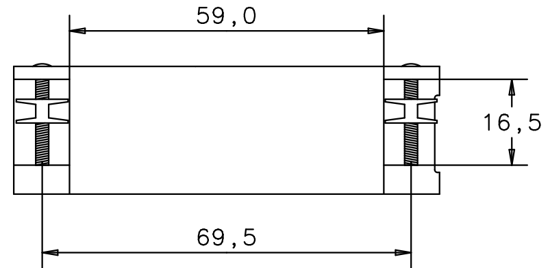
Rückansicht back view
