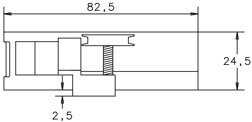
Vorderansicht front view
