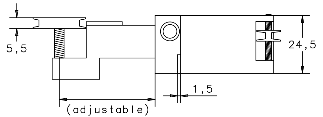
Seitenansicht von rechts side view right
