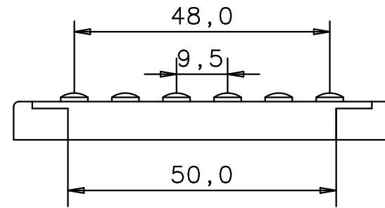
Rückansicht back view
